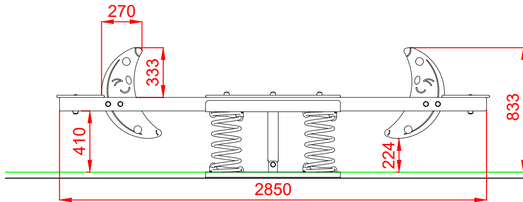
ALZADO
