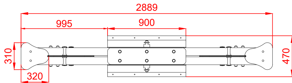
PLANTA
