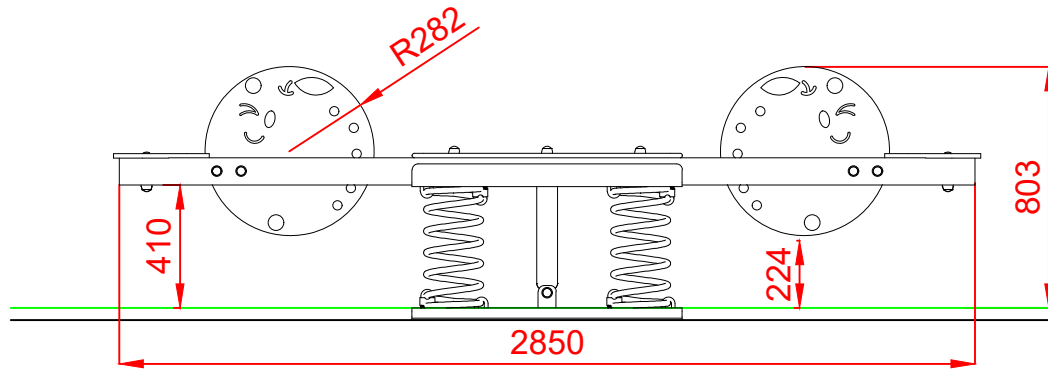
ALZADO
