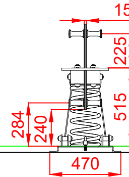
PERFIL
