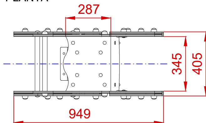
PLANTA
