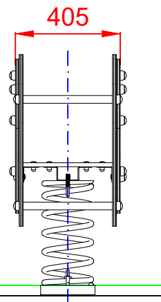
PERFIL
