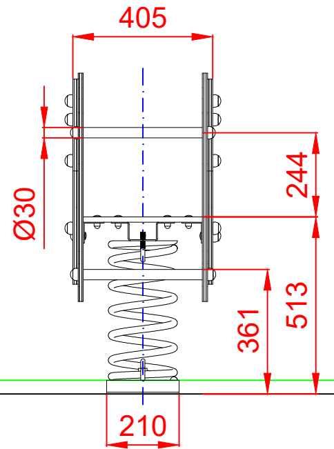
PERFIL
