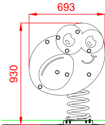
ALZADO
