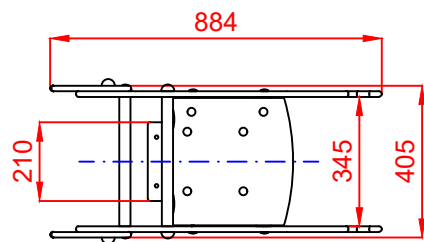
PLANTA
