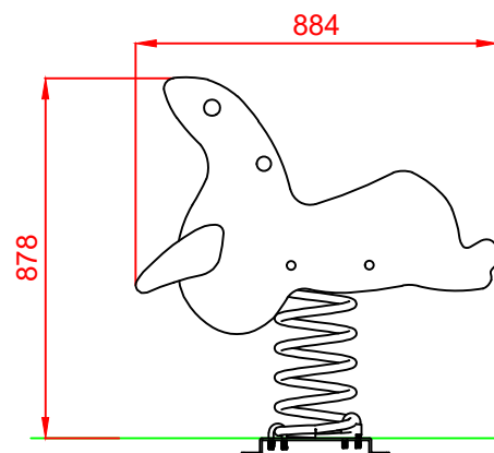
ALZADO
