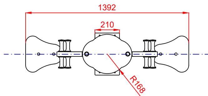
PLANTA
