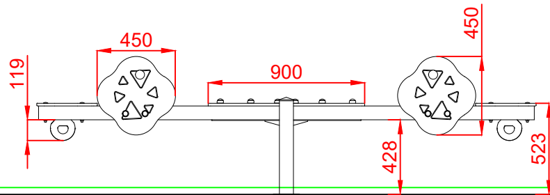
ALZADO
