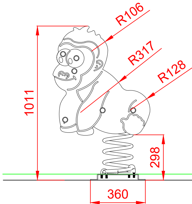
ALZADO
