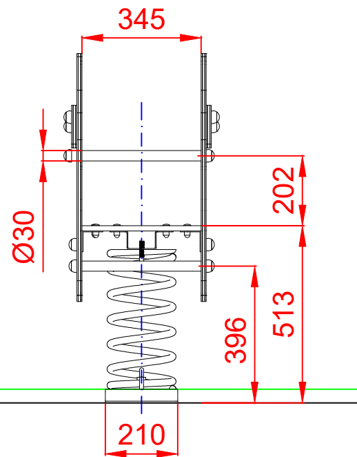
PERFIL
