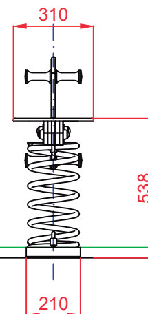
PERFIL
