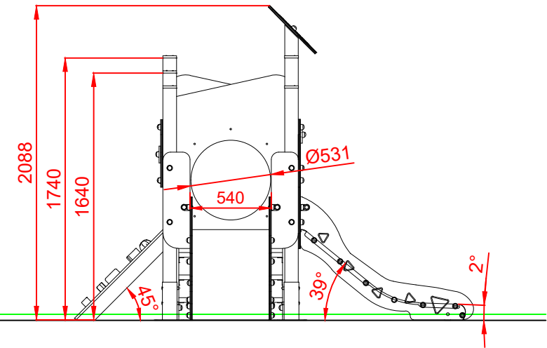
PERFIL IZQUIERDO
