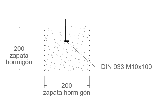
DETALLE ANCLAJE 1:10
