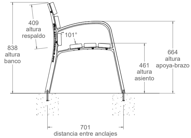
vista lateral 1:20
