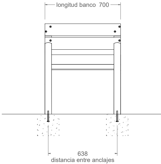
vista frontal 1:20
