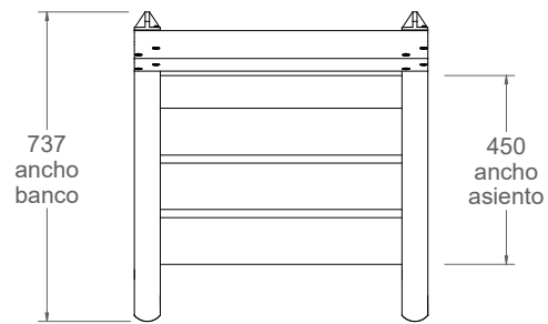
vista en planta 1:20
