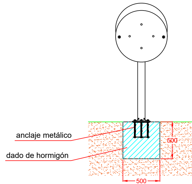
CIMENTACIÓN
