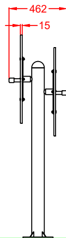
ALZADO
