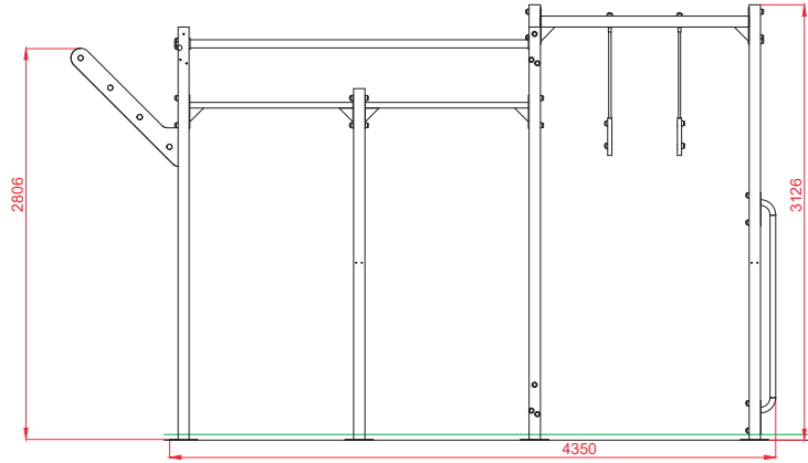
ALZADO
