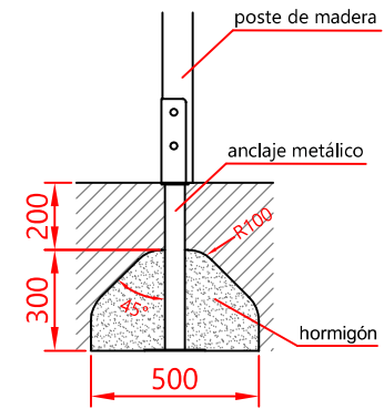
DETALLE DE CIMENTACIÓN HORMIGONADO
