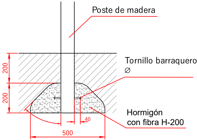
DETALLE DE CIMENTACIÓN HORMIGONADO E=2/1
