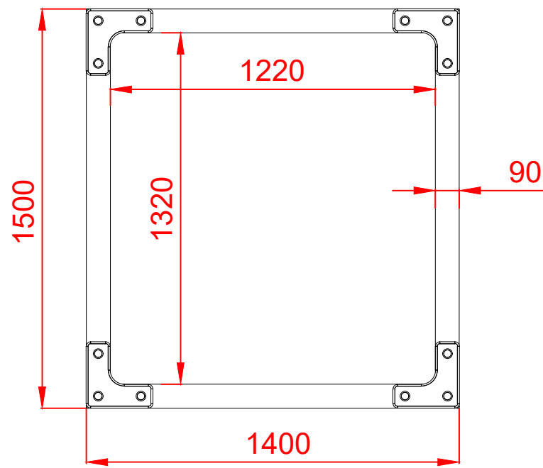
PLANTA
