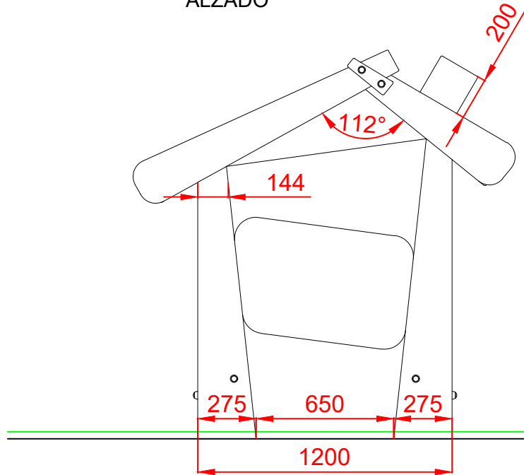
ALZADO
