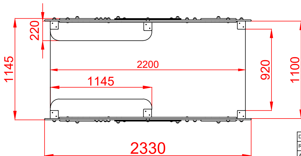
PLANTA
