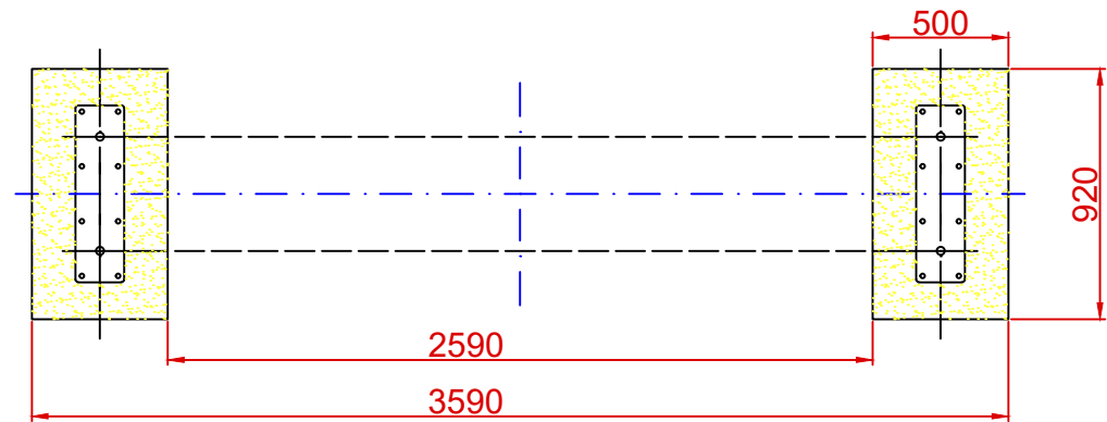
PLANTA CIMENTACIÓN
