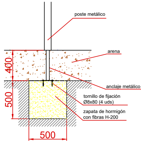
ESQUEMA DE CIMENTACIÓN EN ARENA
