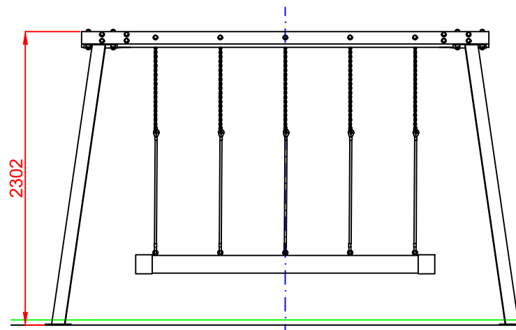
ALZADO
