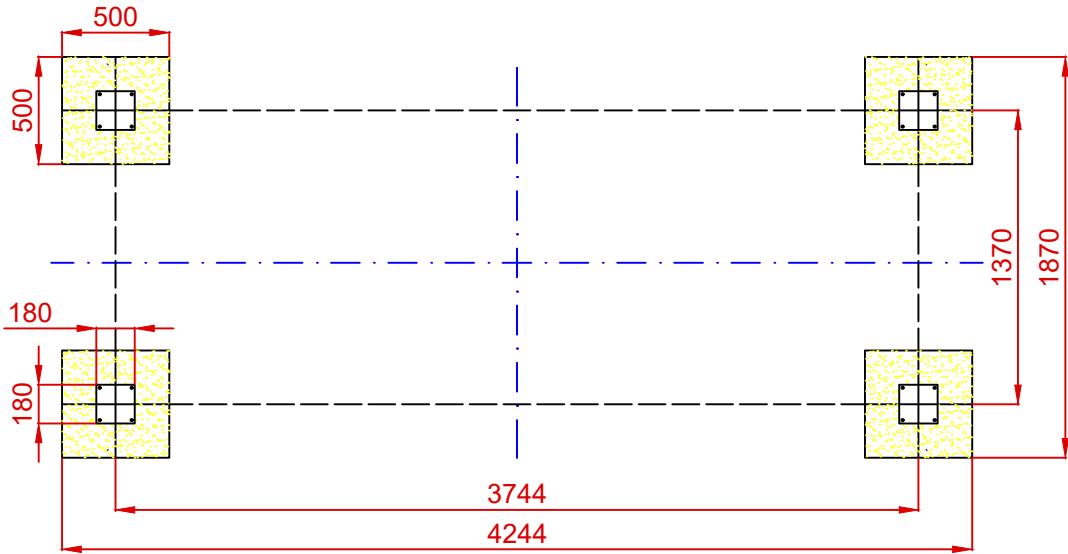
PLANTA CIMENTACIÓN
