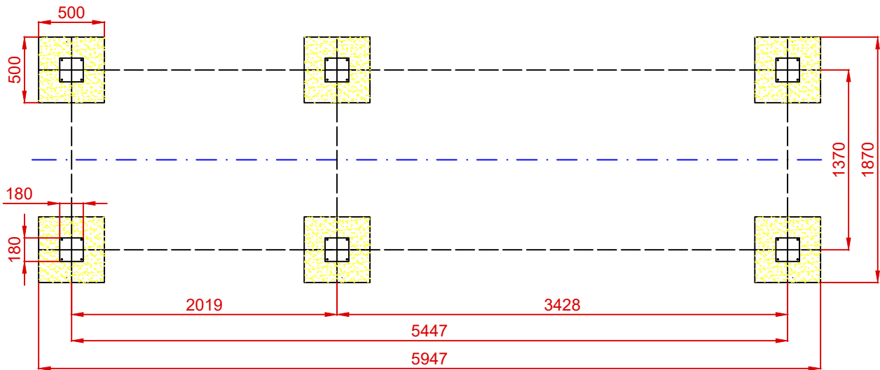
PLANTA CIMENTACIÓN
