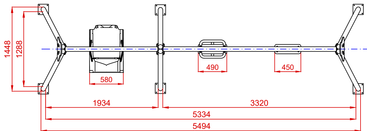
PLANTA
