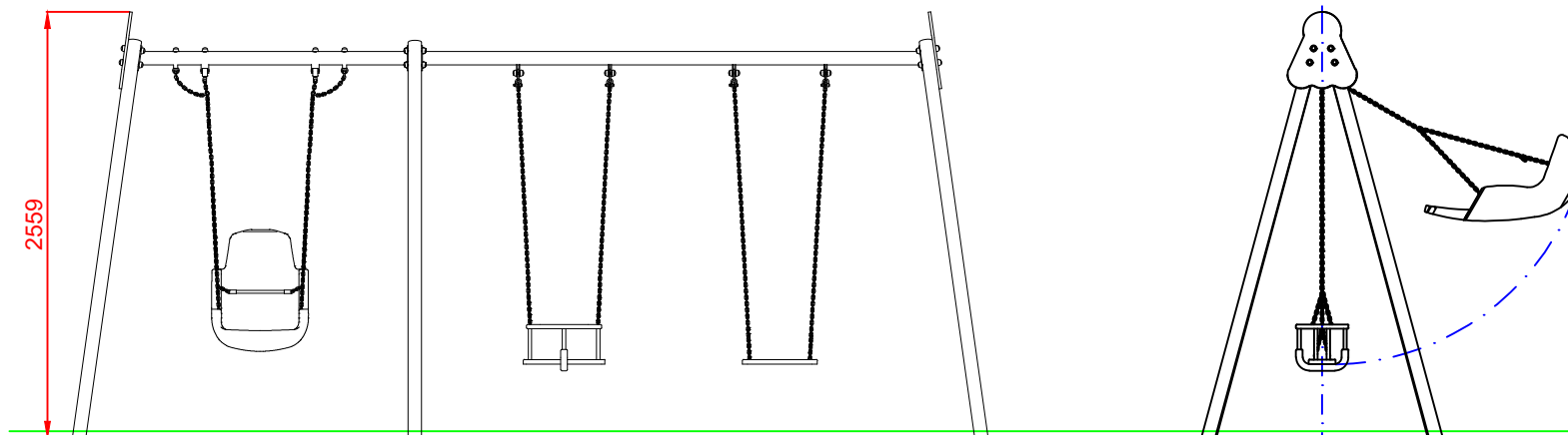
ALZADO
