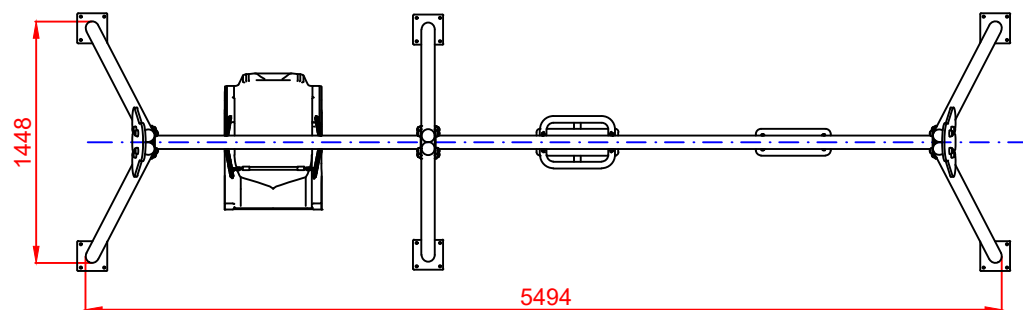
PLANTA
