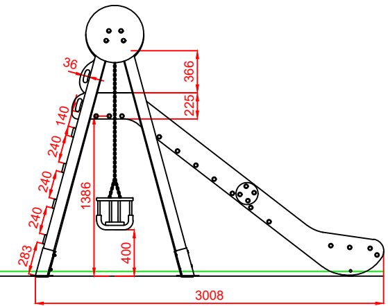
PERFIL IZQUIERDO
