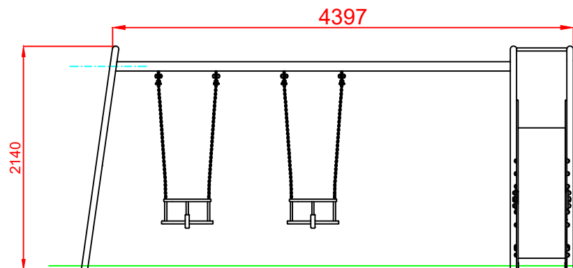
ALZADO
