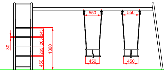
ALZADO POSTERIOR
