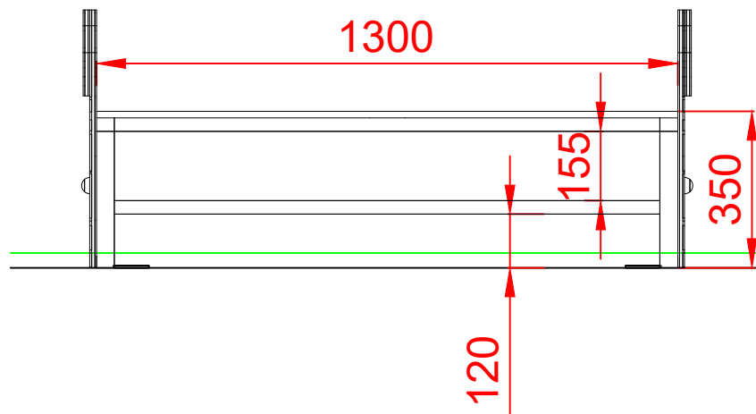
ALZADO
