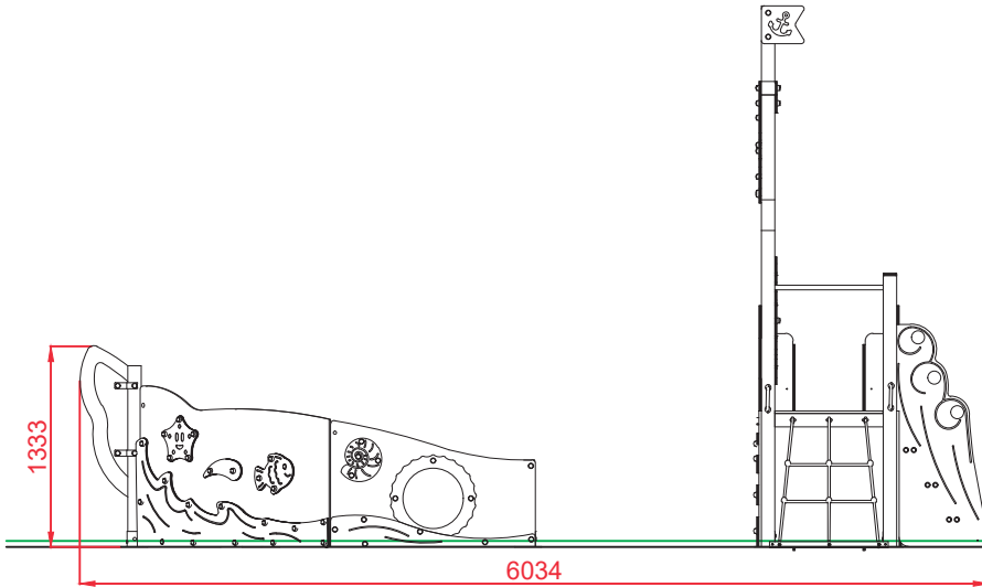
ALZADO
