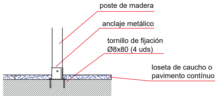
ESQUEMA DE CIMENTACIÓN EN HORMIGÓN E: 2/1
