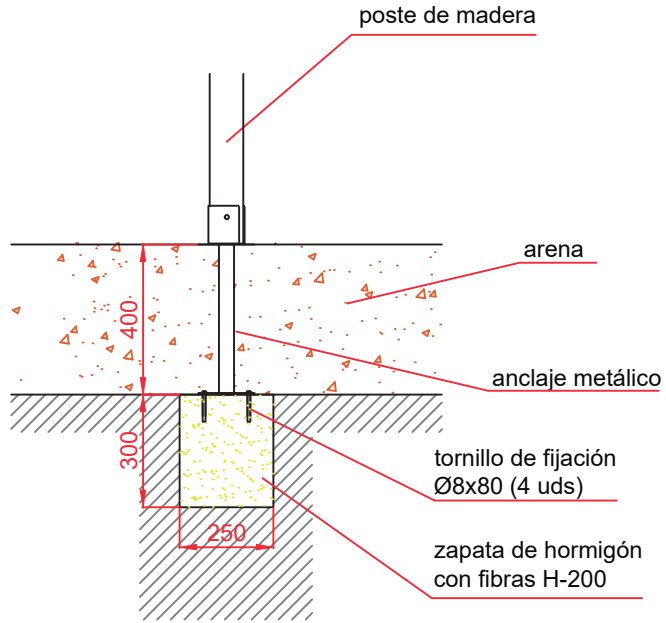
ESQUEMA DE CIMENTACIÓN EN ARENA E: 2/1
