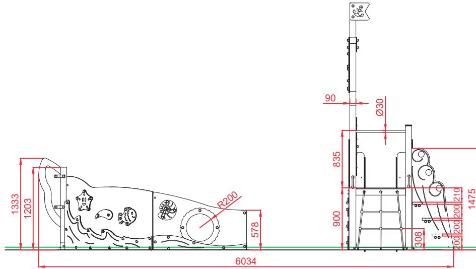
ALZADO
