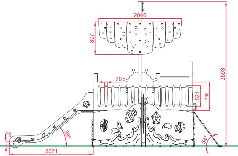
PERFIL IZQUIERDO
