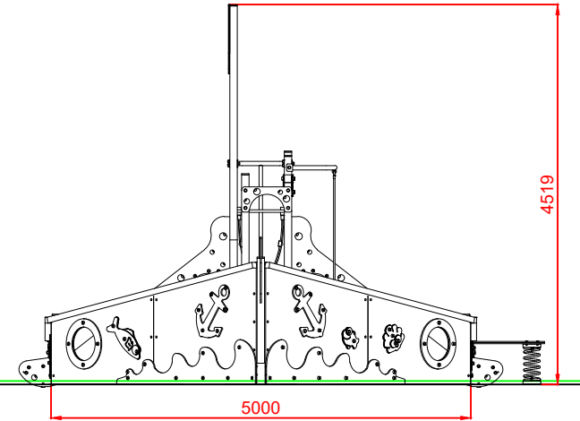
PERFIL IZQUIERDO
