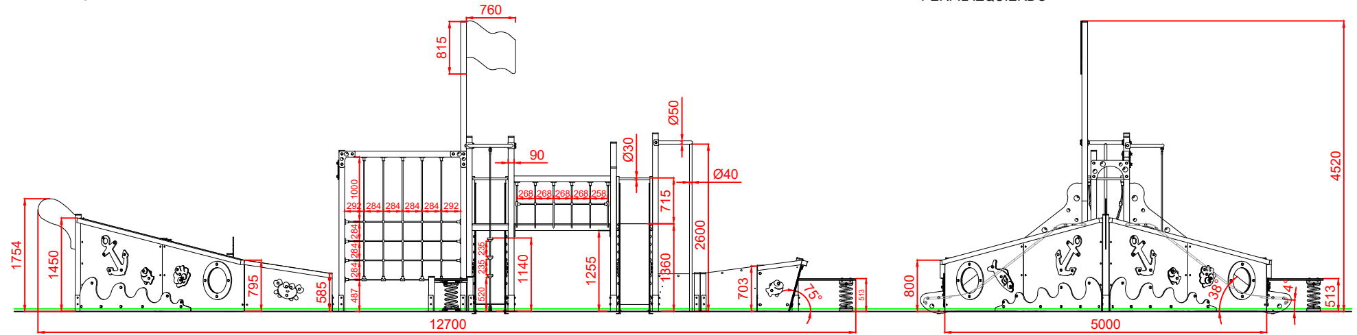
ALZADO
