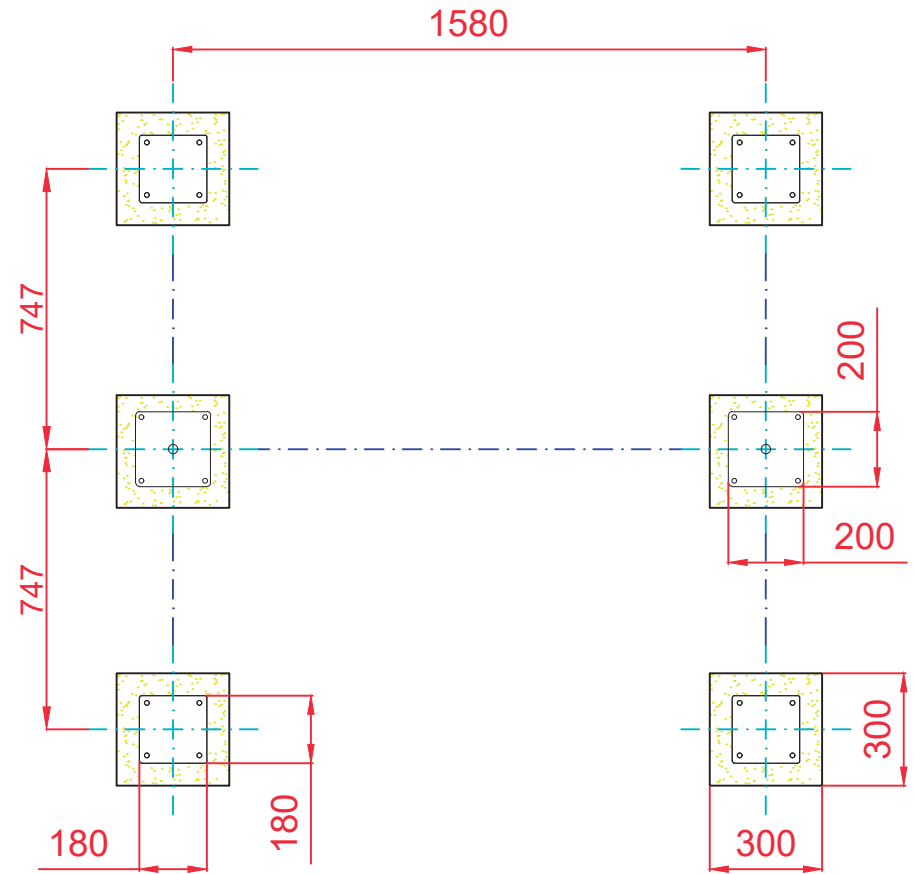
PLANTA
