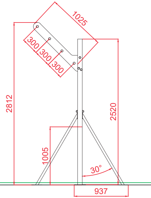
PERFIL
