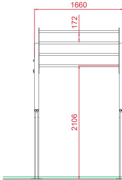
ALZADO
