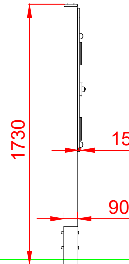
PERFIL IZQUIERDO
