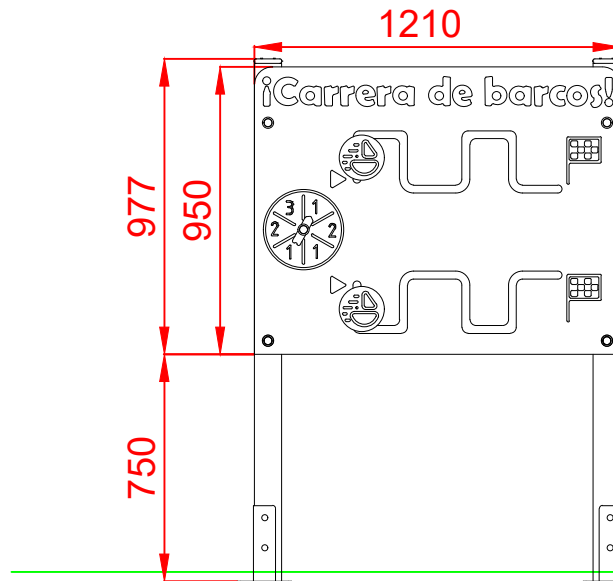
ALZADO
