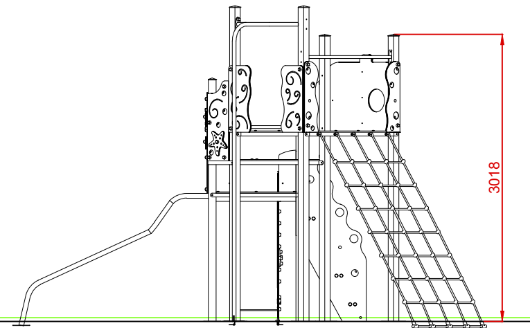
PERFIL IZQUIERDO
