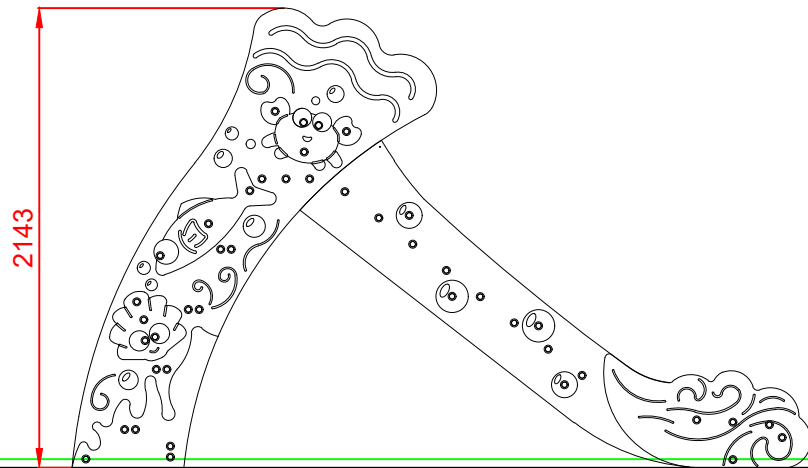
ALZADO
