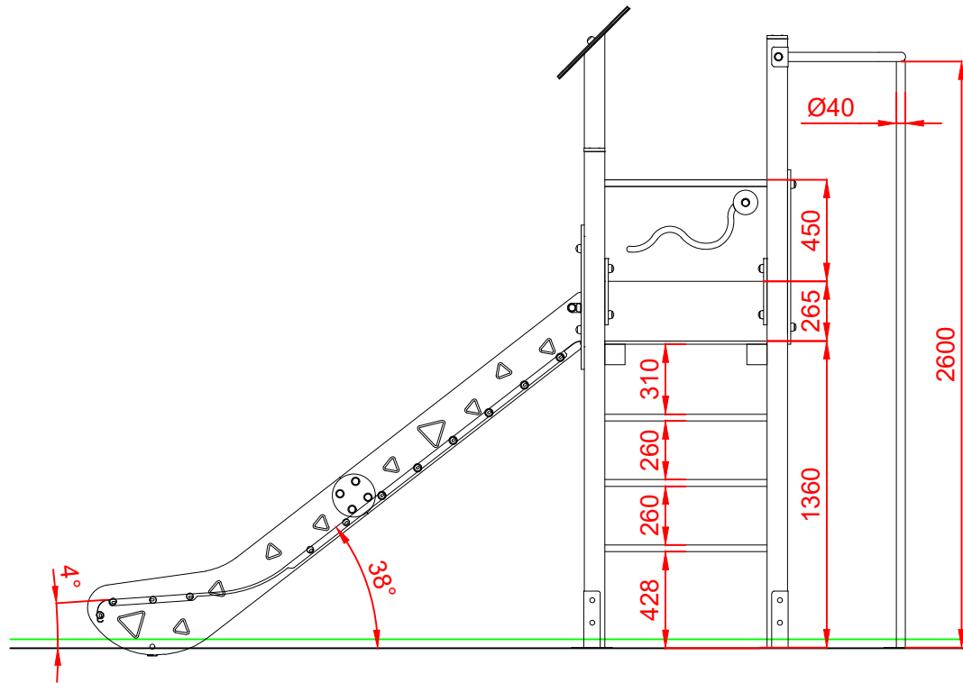
ALZADO
