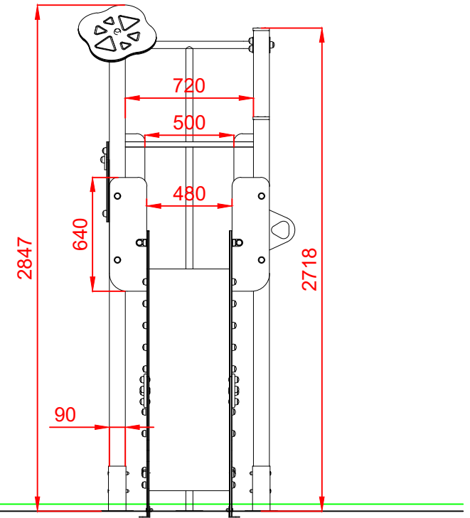
PERFIL IZQUIERDO
