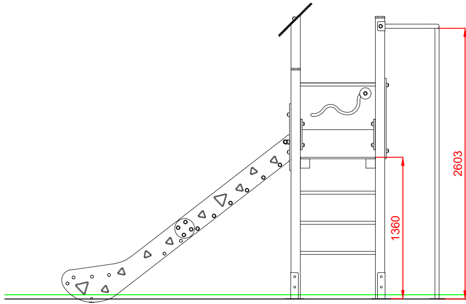
ALZADO
