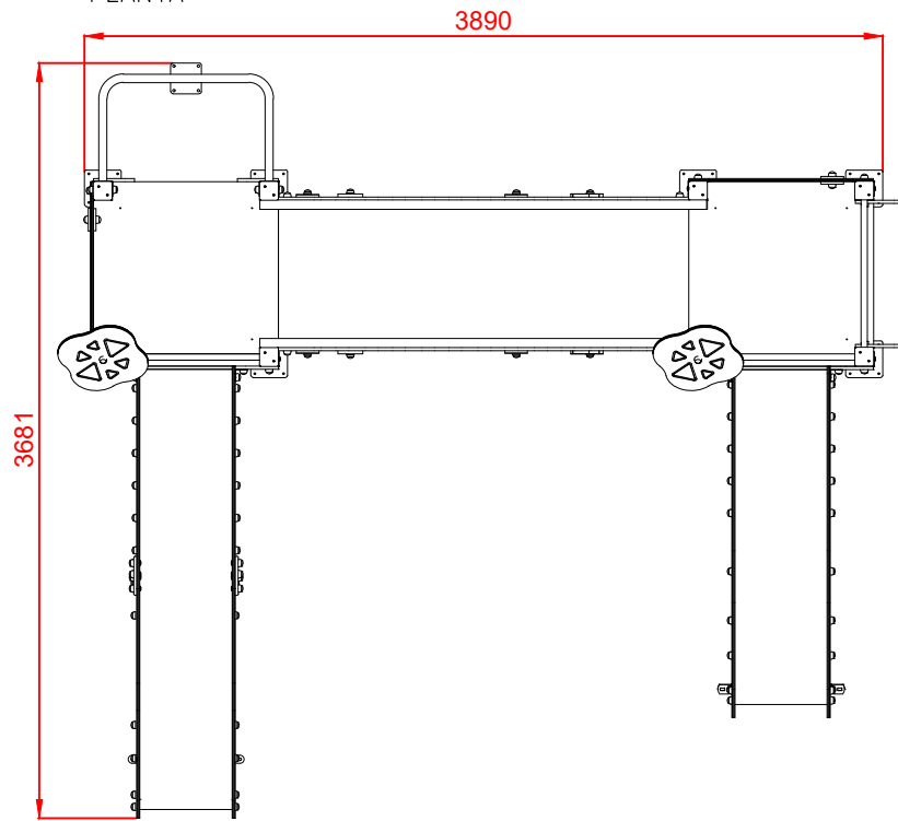
PLANTA
