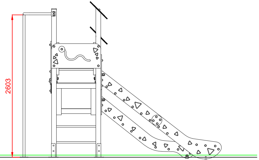
PERFIL IZQUIERDO
