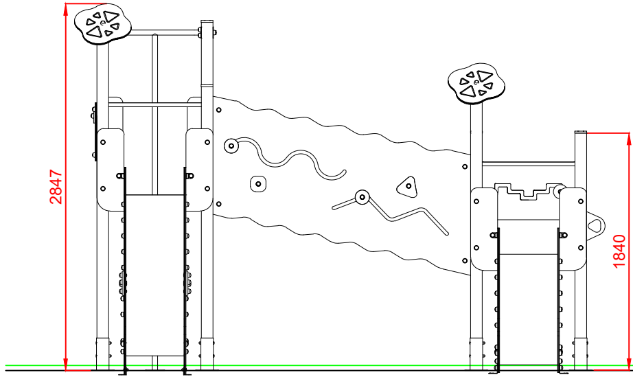
ALZADO
