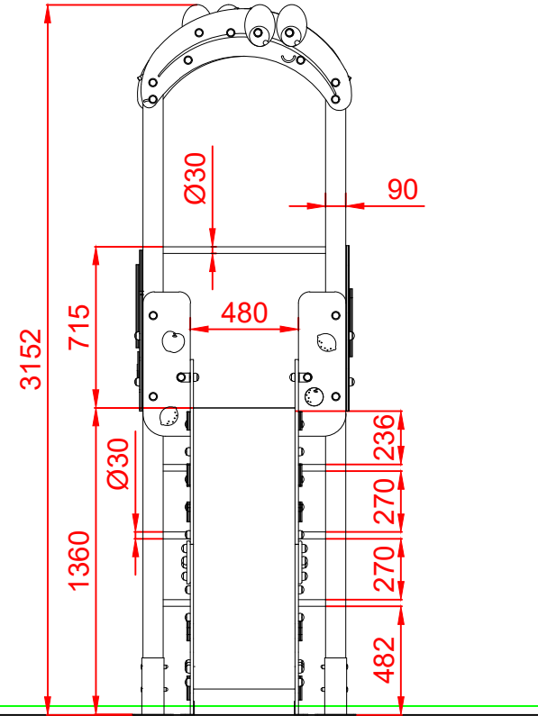
PERFIL IZQUIERDO
