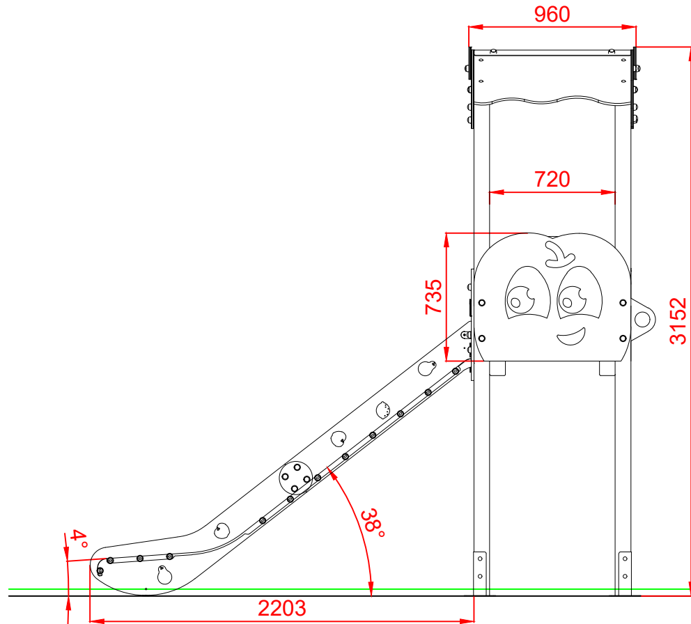
ALZADO
