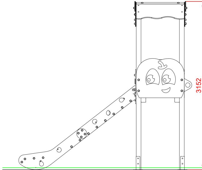
ALZADO
