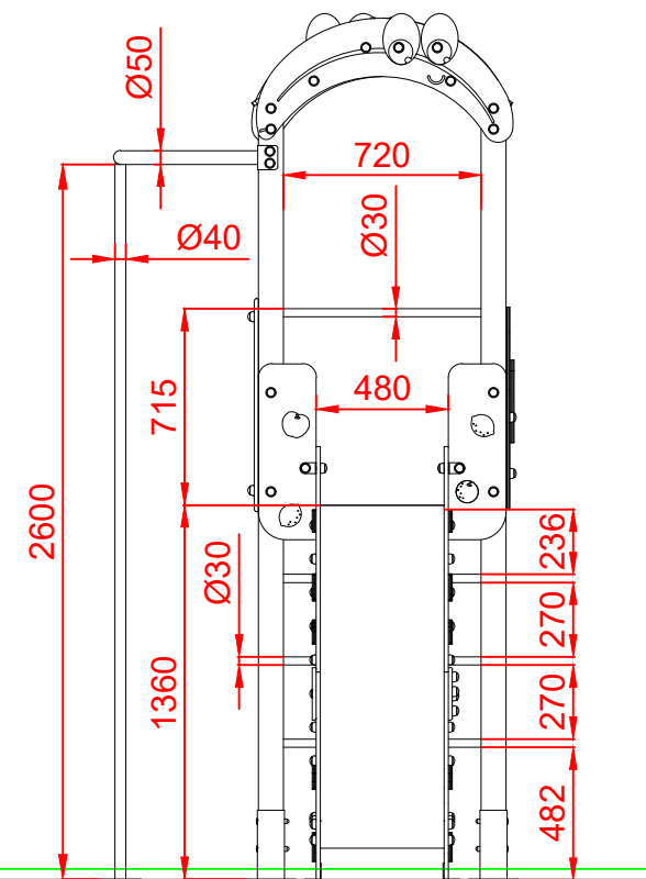
PERFIL IZQUIERDO
