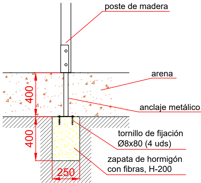
ESQUEMA DE CIMENTACIÓN EN ARENA
