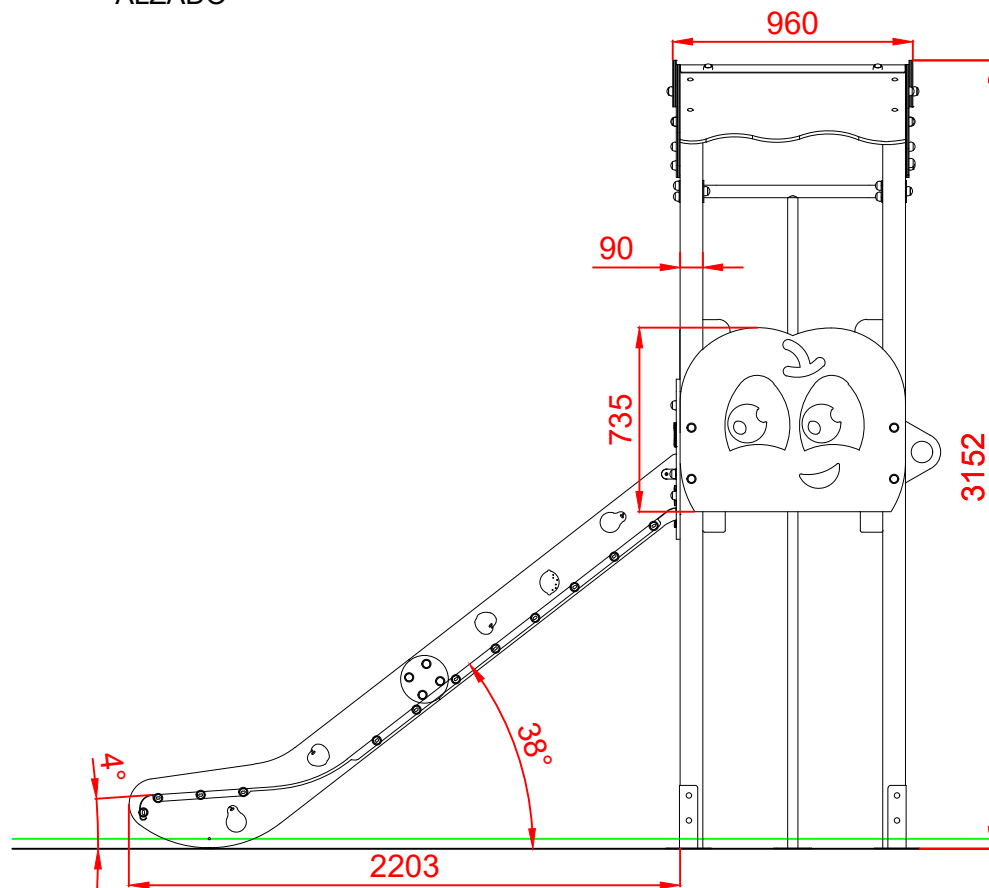
ALZADO
