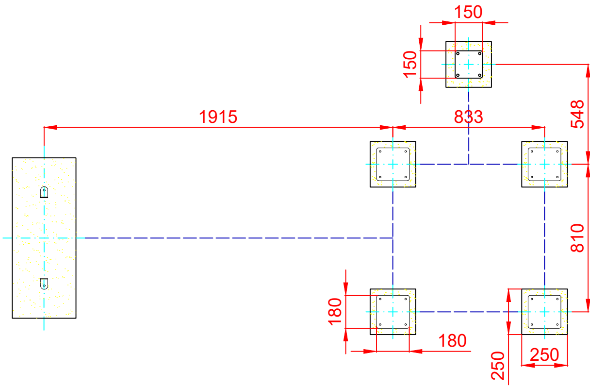
PLANTA CIMENTACIÓN
