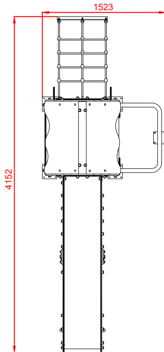
PLANTA
