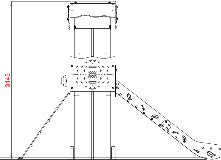
PERFIL IZQUIERDO
