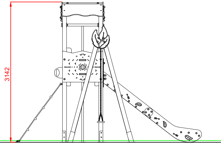
PERFIL IZQUIERDO
