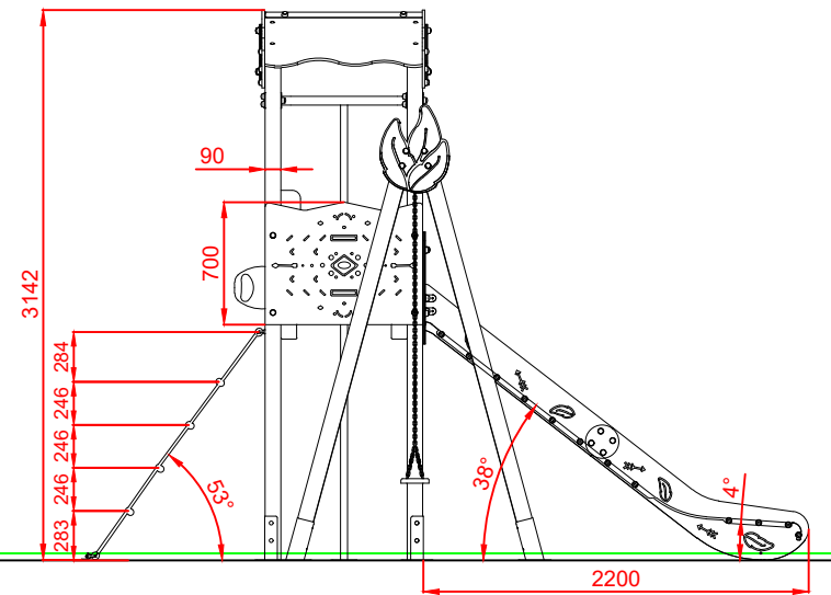
PERFIL IZQUIERDO
