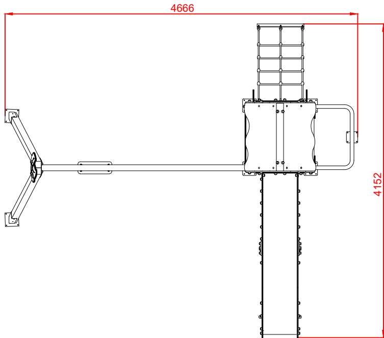
PLANTA
