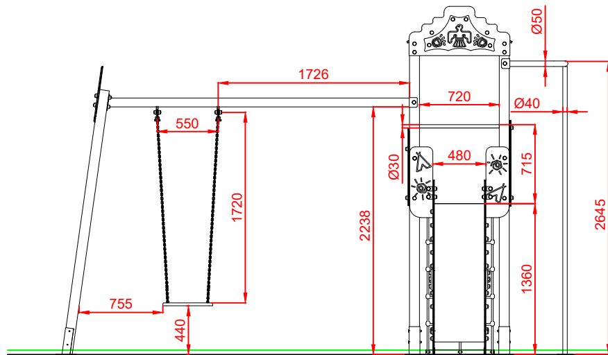
ALZADO
