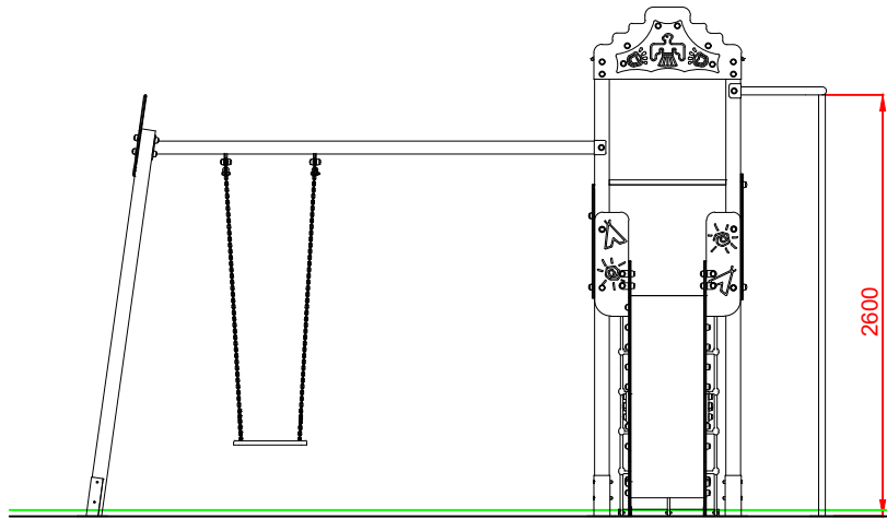
ALZADO
