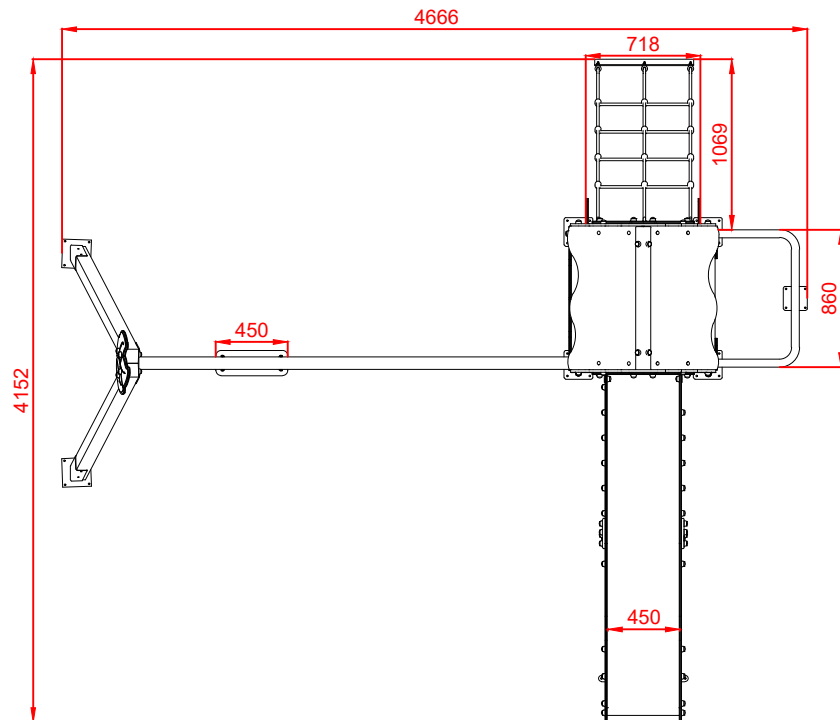
PLANTA
