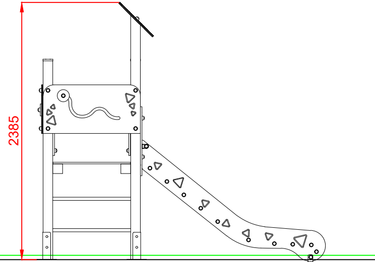
PERFIL IZQUIERDO
