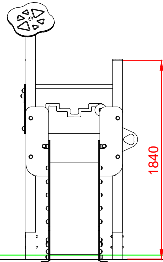
ALZADO
