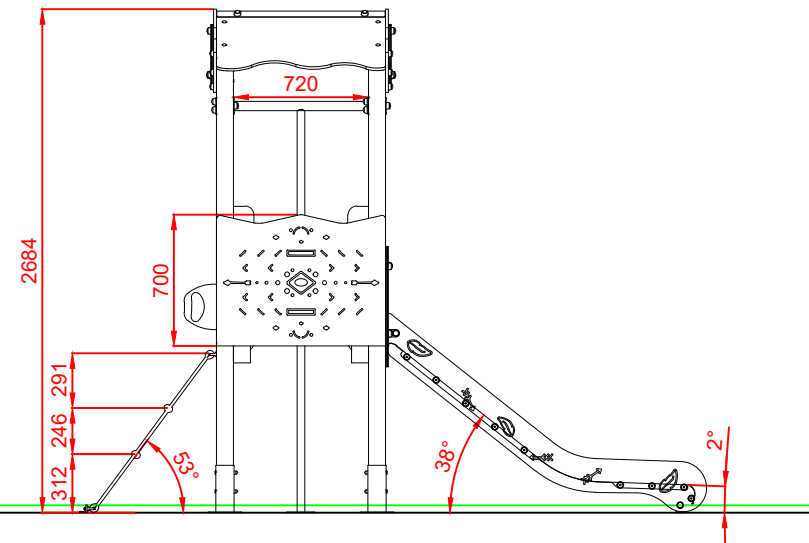
PERFIL IZQUIERDO
