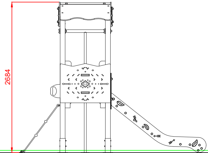
PERFIL IZQUIERDO
