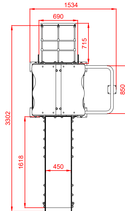
PLANTA
