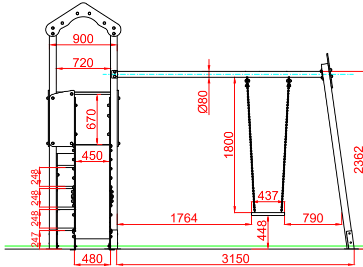
ALZADO
