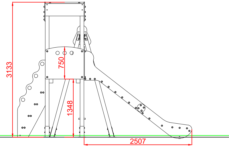
PERFIL IZQUIERDO
