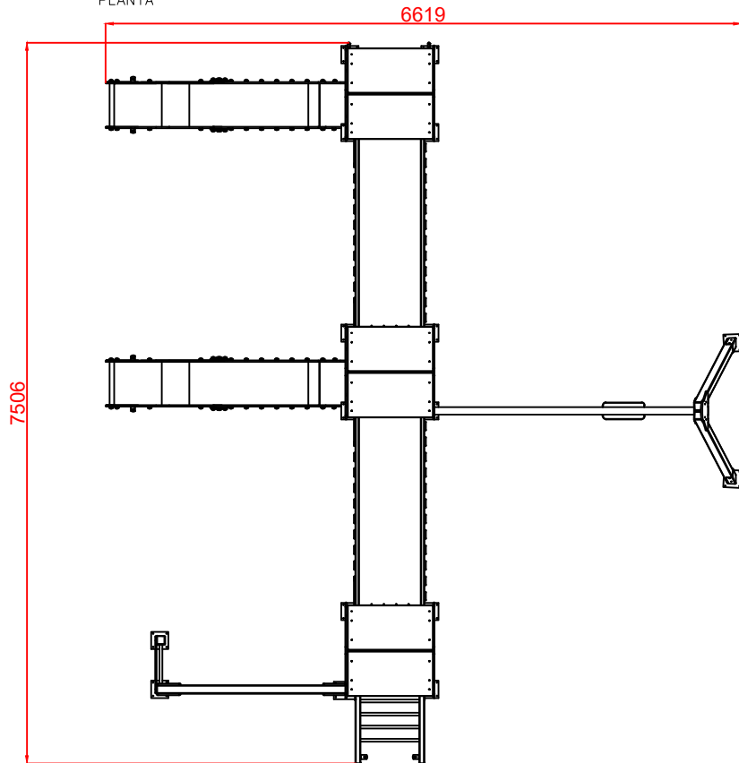
PLANTA
