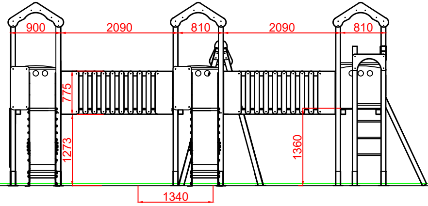
PERFIL IZQUIERDO
