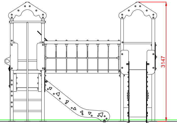
PERFIL IZQUIERDO
