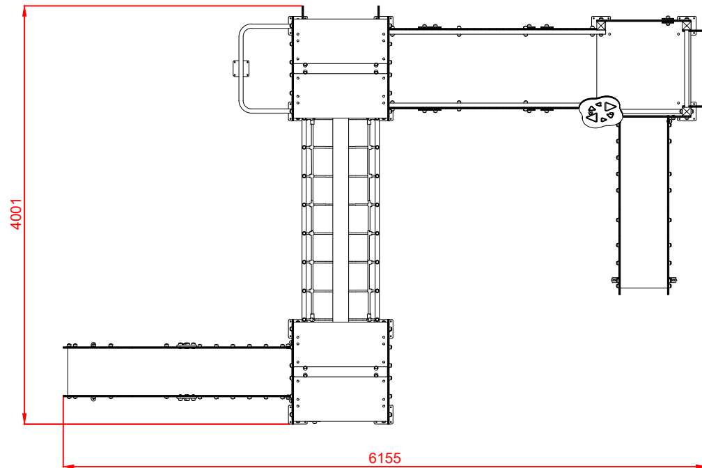
PLANTA
