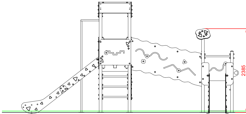
ALZADO
