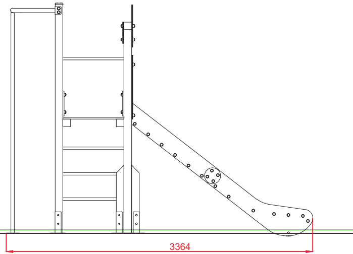
PERFIL IZQUIERDO
