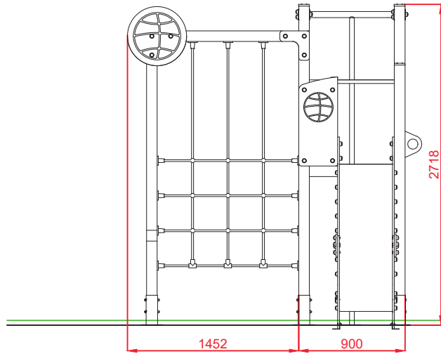
ALZADO
