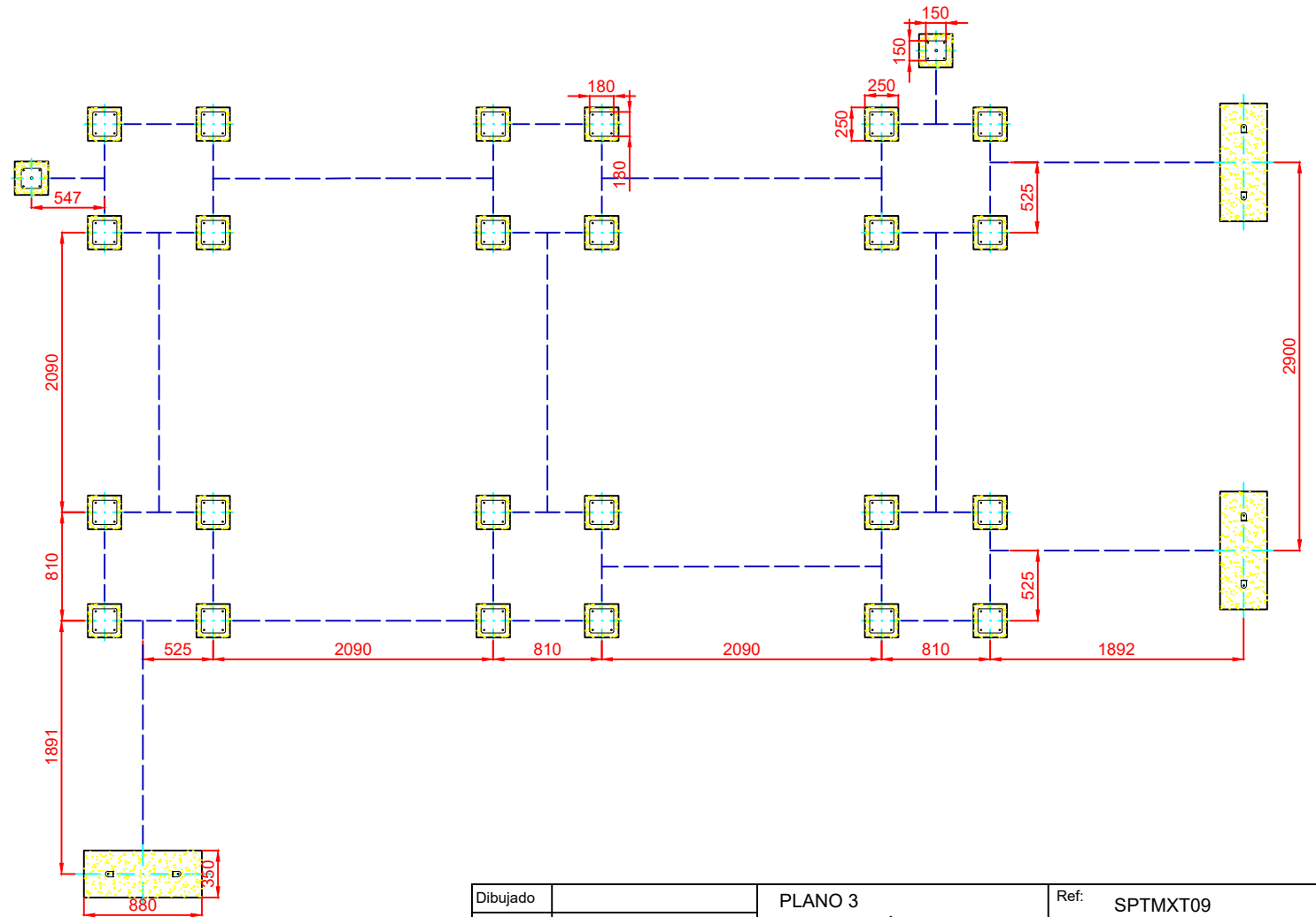
PLANTA CIMENTACIÓN
