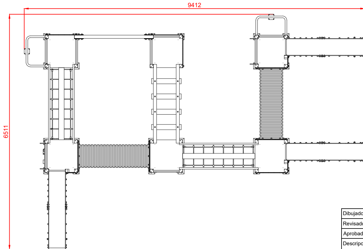
PLANTA
