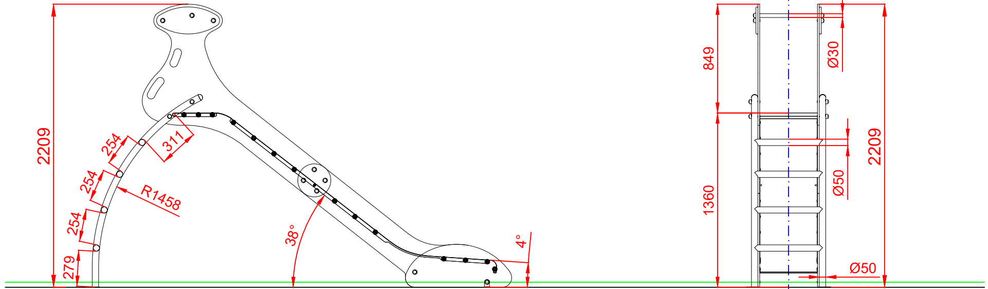
ALZADO
