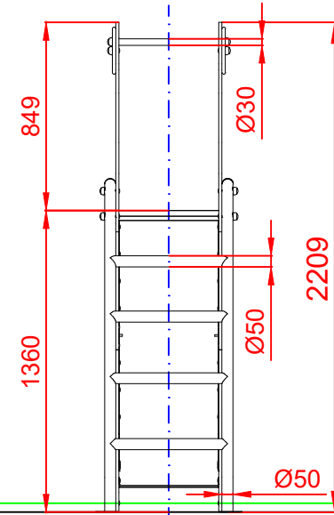
PERFIL IZQUIERDO
