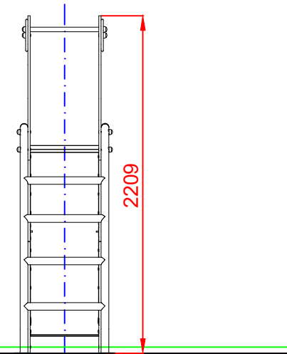
PERFIL IZQUIERDO
