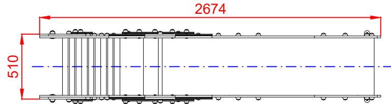
PLANTA
