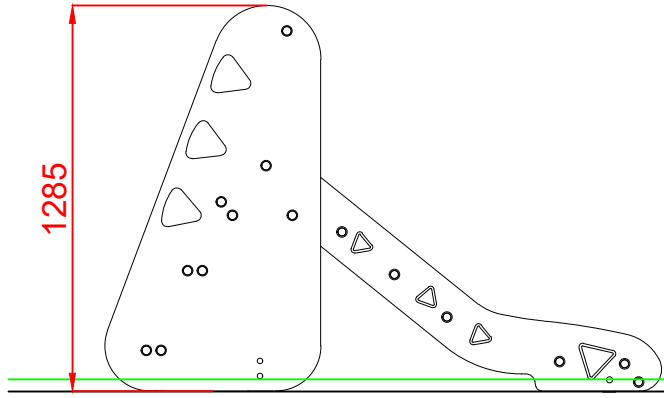
ALZADO
