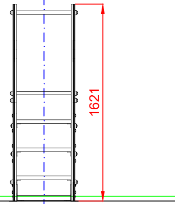
PERFIL IZQUIERDO
