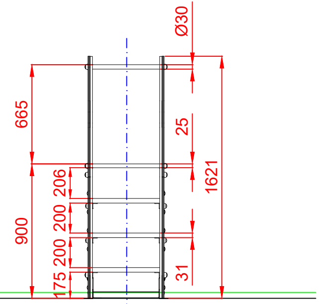
PERFIL IZQUIERDO
