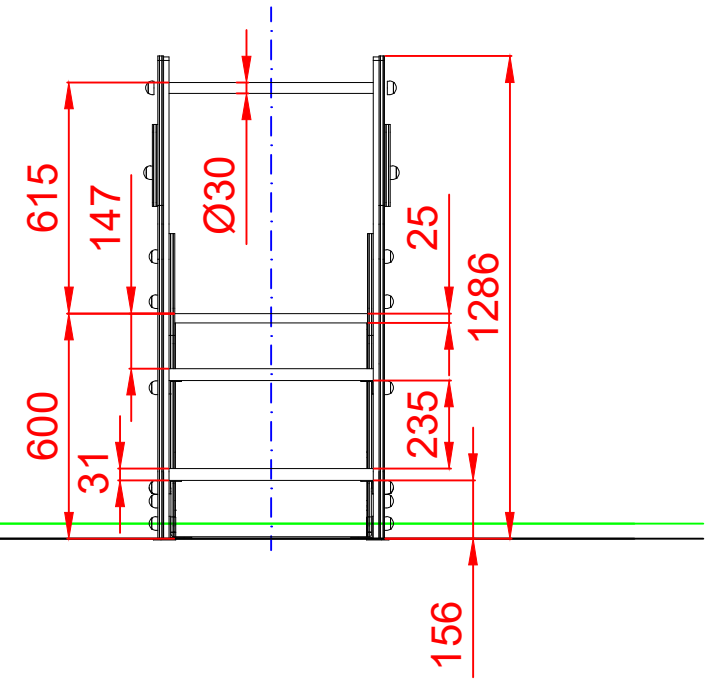
PERFIL IZQUIERDO
