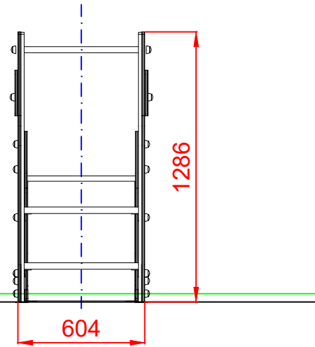
PERFIL IZQUIERDO
