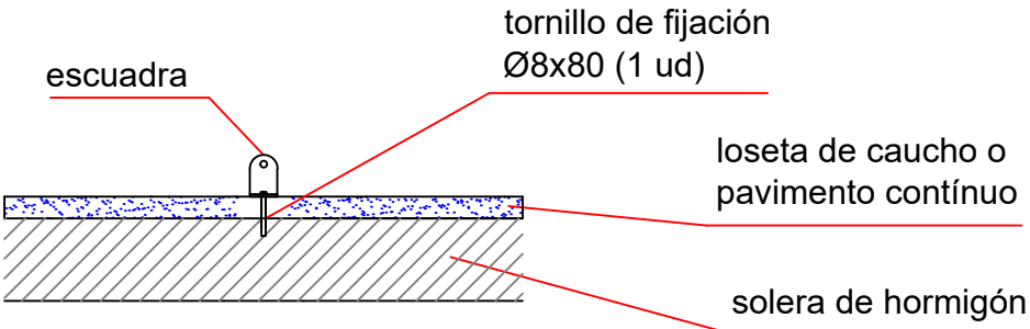
ESQUEMA DE CIMENTACIÓN EN HORMIGÓN E: 2/1
