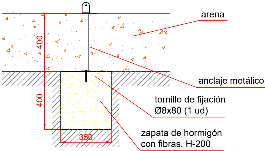
ESQUEMA DE CIMENTACIÓN EN ARENA E: 2/1
