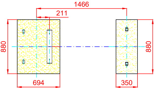
PLANTA CIMENTACIÓN
